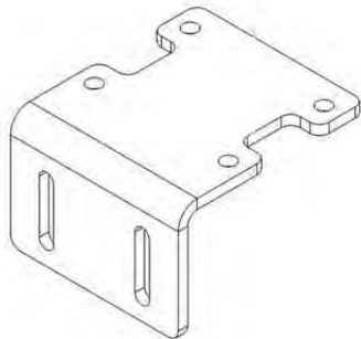
110-170191-001 2 REQD
